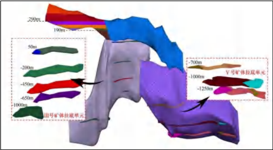
图 5-2-38 多矿体协同开采全过程数值模拟顺序图
