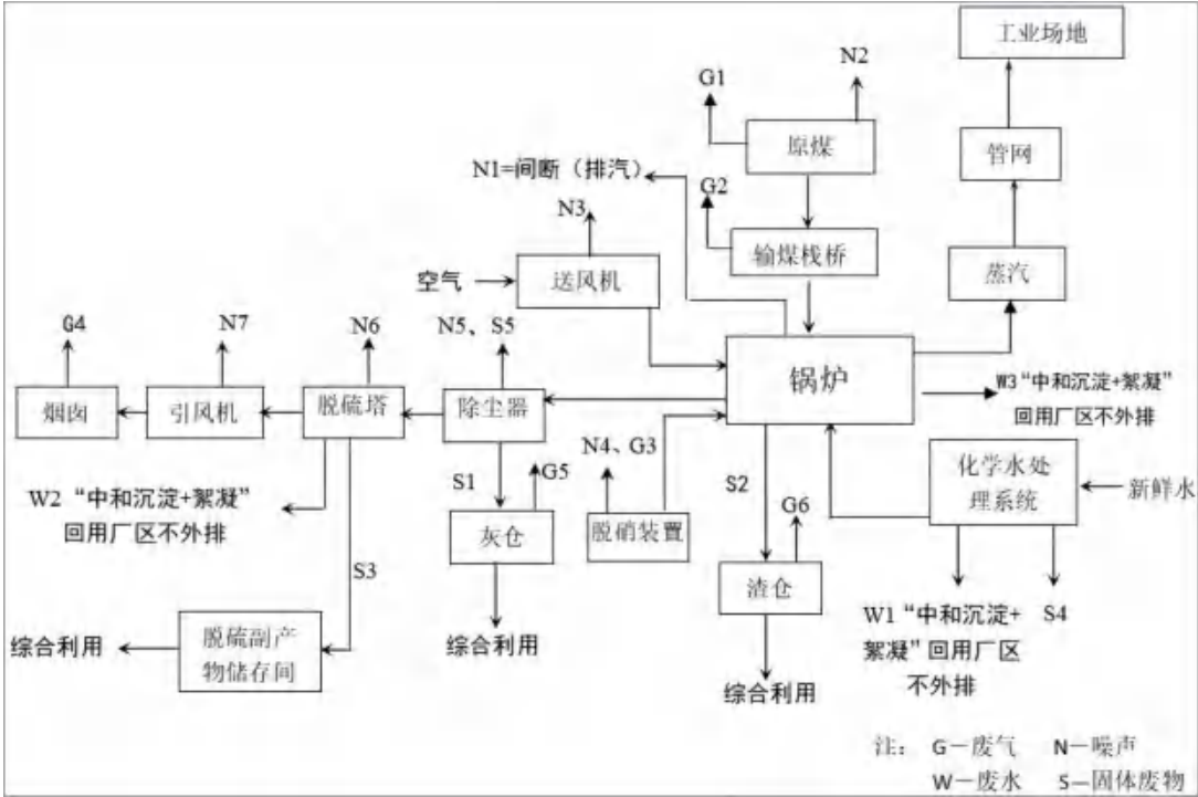
图 3-3-3 供热工程工艺流程及产污节点图
