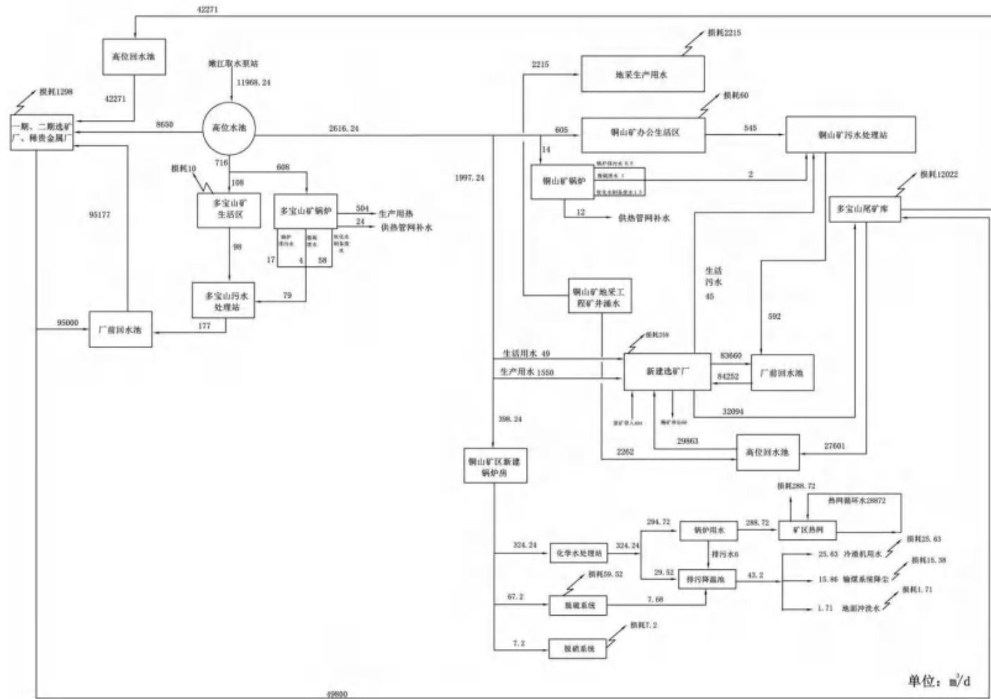
图 3-2-7 一期工程建成后矿区冬季水量平衡图
