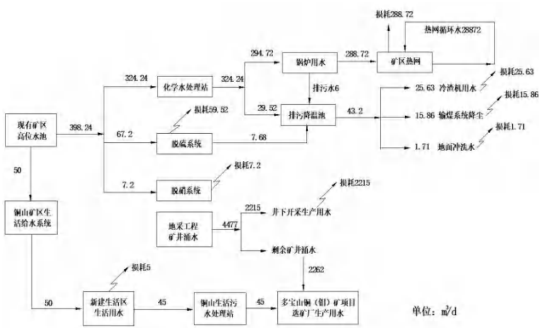
图 3-2-5 本项目一期工程冬季水量平衡图
