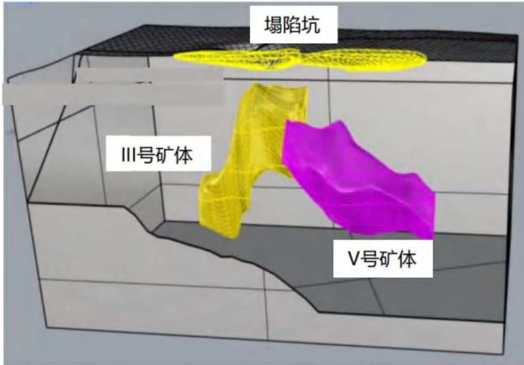
图 5-2-52 III、V 号矿体最终塌陷坑形态示意图
