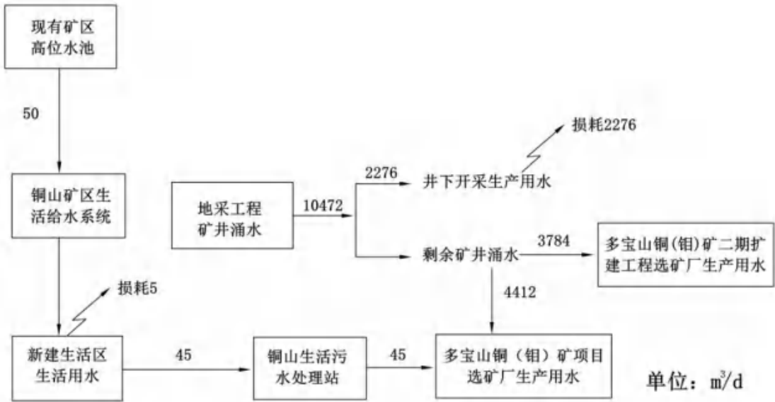
图 3-2-8 本项目二期工程夏季水量平衡图
