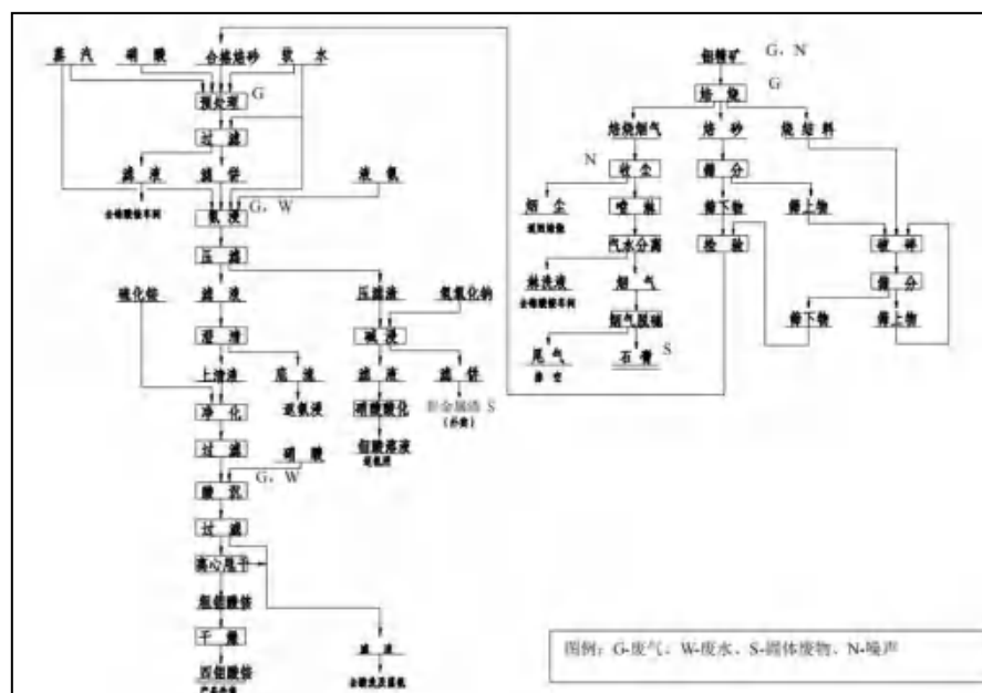
图 3-1-10 钼精矿综合回收利用工程生产工艺流程图
