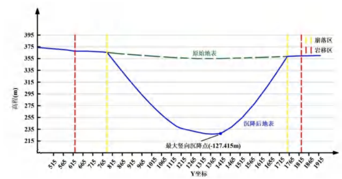
图 5-2-51 V号矿体开采前后地表高程变化示意图
