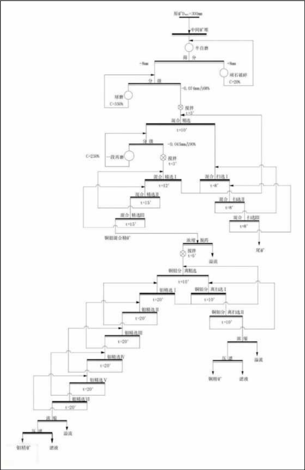
图 3-1-20 选矿生产工艺流程图
