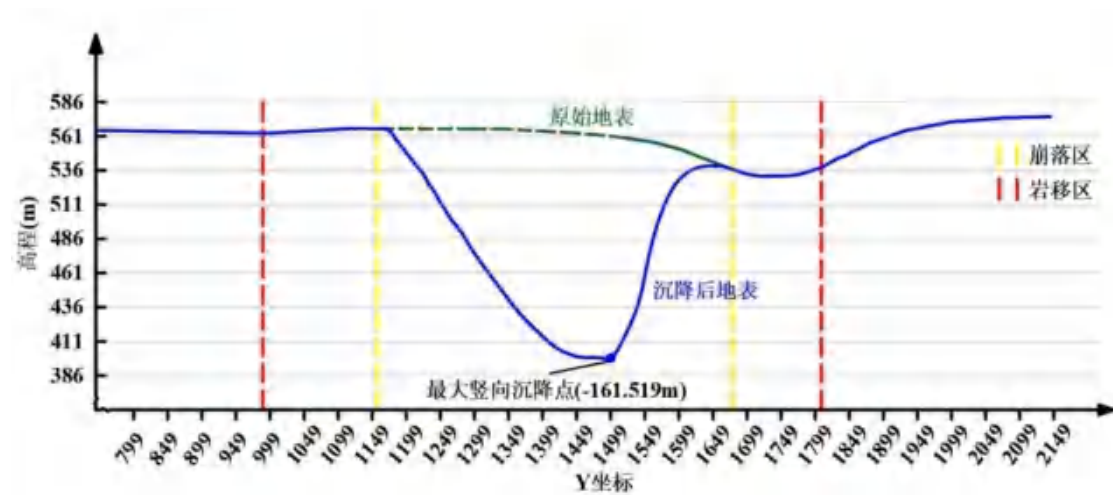
图 5-2-50 III号矿体开采前后地表高程变化示意图
