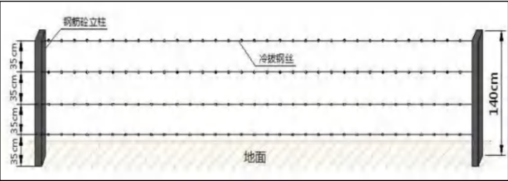
图 6-2-4 铁丝防护栏示意图
