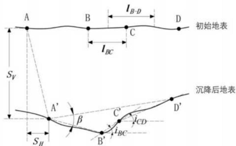
图 5-2-39 沉降前后的地表特征点示意图
