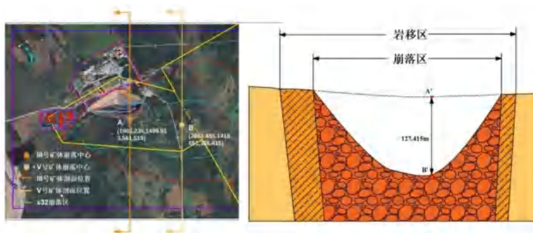
图 5-2-49 沿矿体走向 V 号矿体塌陷坑中心剖面图
