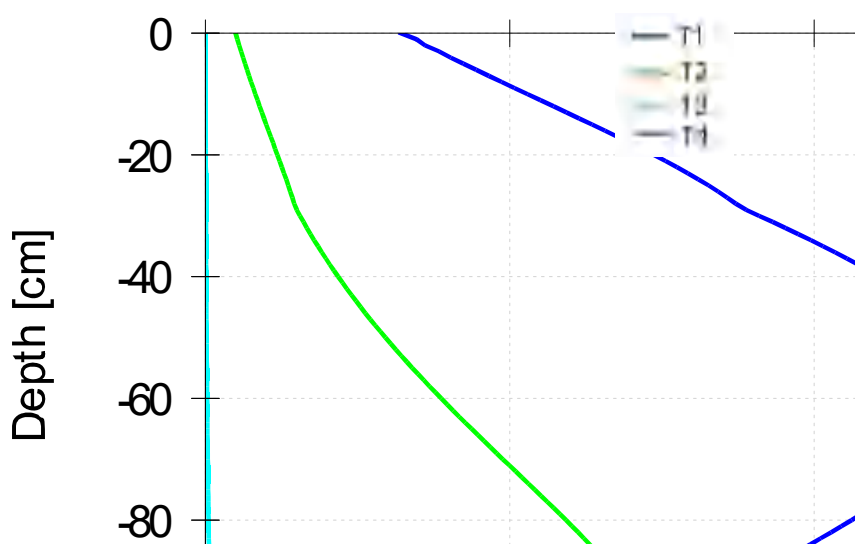
图5-2-29 铅垂向运移情况图
