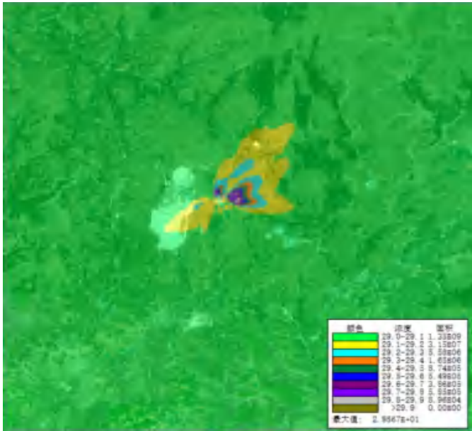
图 5-2-5 本项目 PM 2.5 保证率日平均质量浓度分布图 (ug/m 3 )
