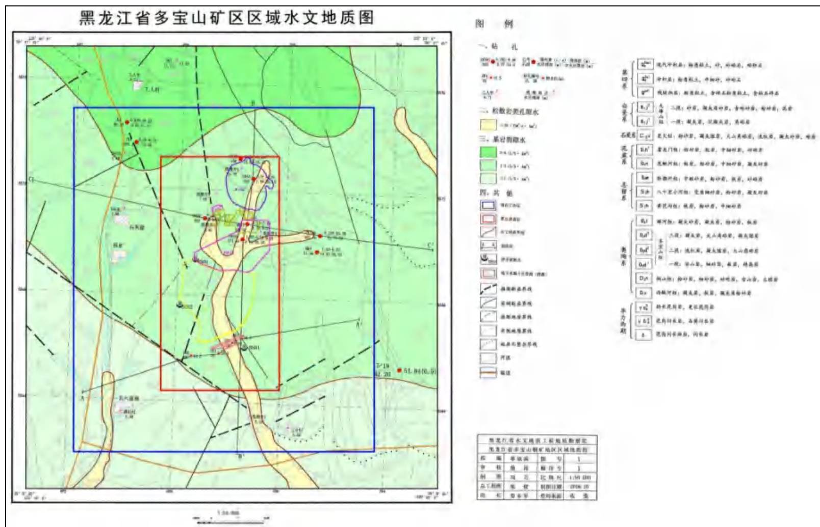
图 4-1-4 区域水文地质图
