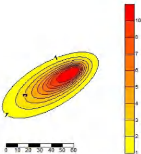
图 5-2-21 非正常状况下氟化物污染晕扩散预测图 (1000d)
