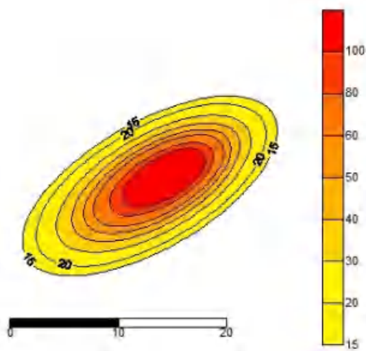
5-2-17 非正常状况下 COD 扩散预测图（100d）
