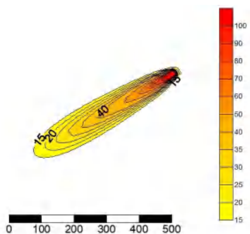
图 5-2-19 非正常状况下 COD 污染晕扩散预测图 (34a)
