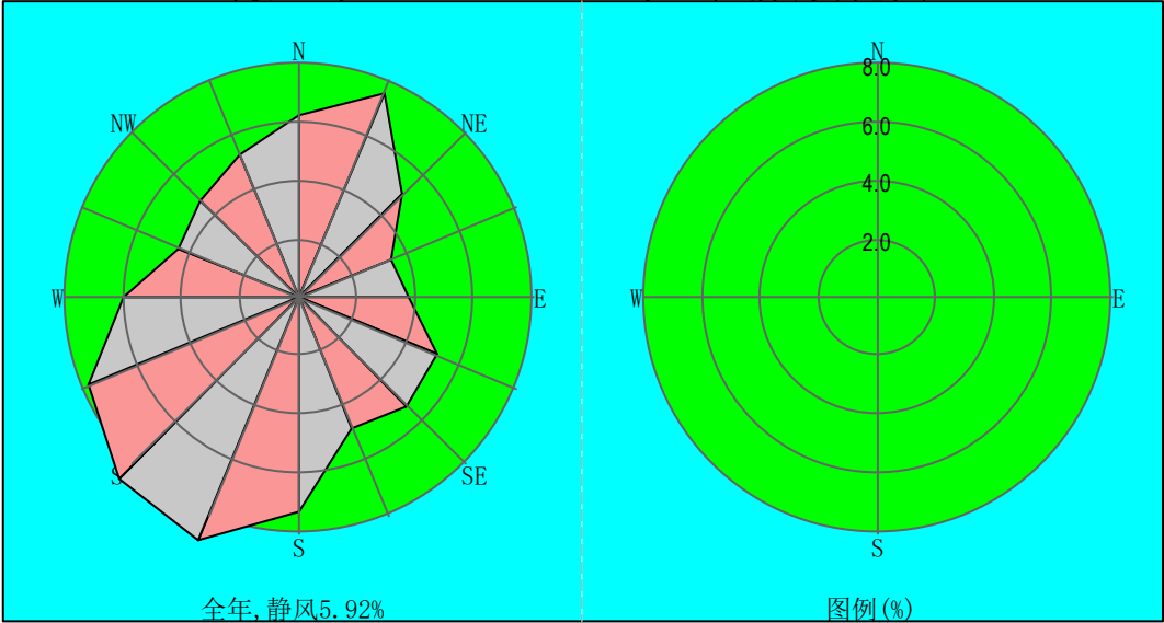
嫩江市（2003-2022年）风频玫瑰图
