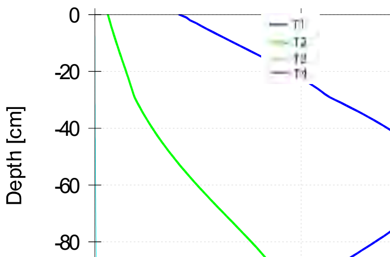
图5-2-33 砷垂向迁移情况图
