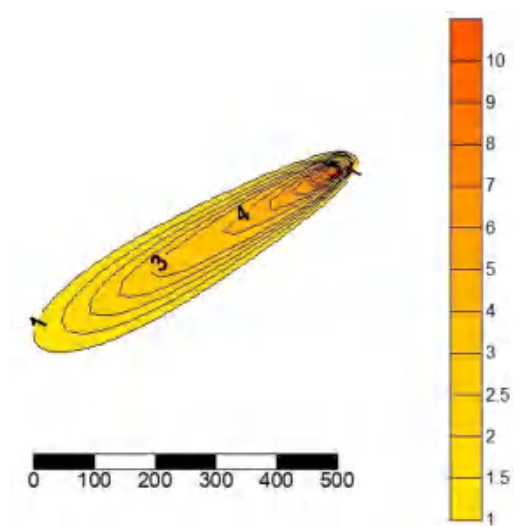
图 5-2-22 非正常状况下氟化物扩散预测图（30a）
