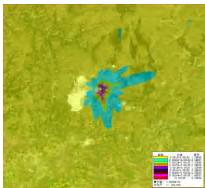
图 5-2-10 本项目 TSP 日平均质量浓度分布图 (ug/m³)
