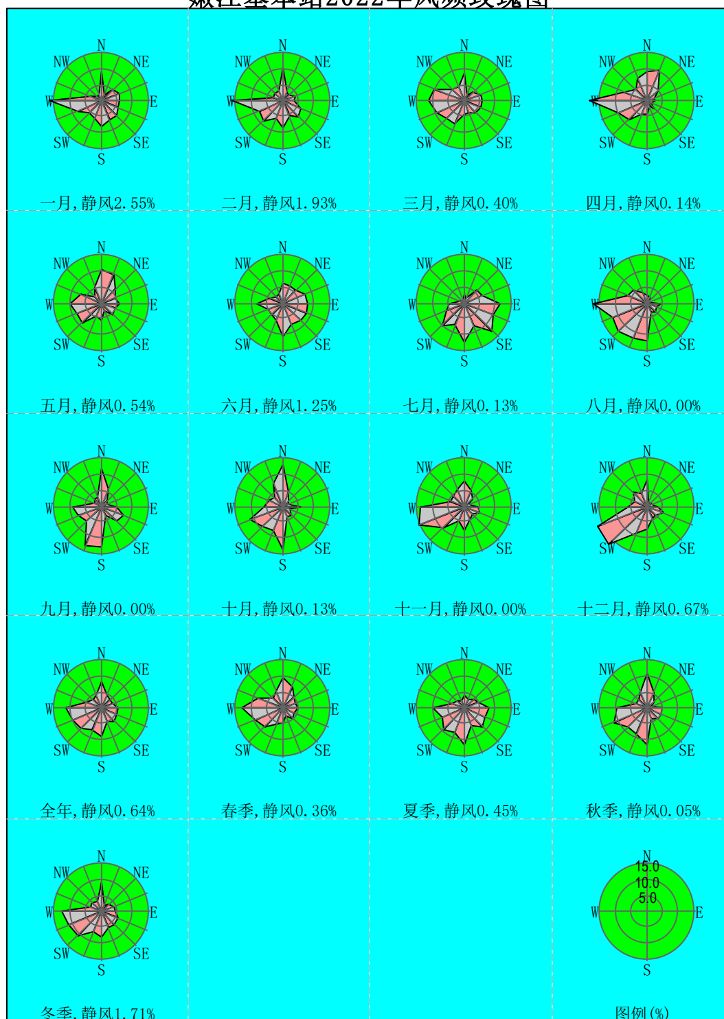
图 4-1-10 嫩江市 2022 年年风频玫瑰图
