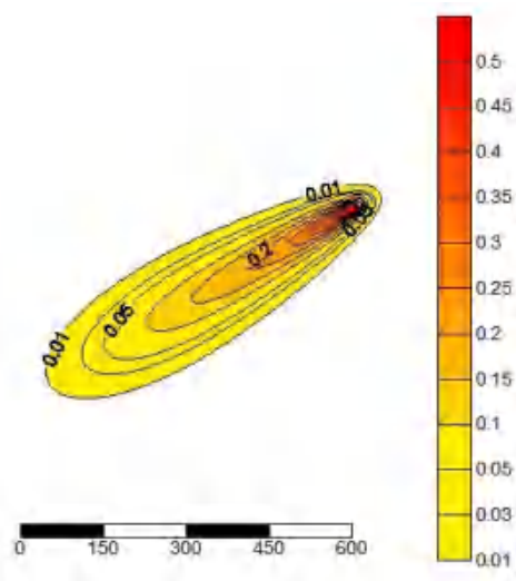
图 5-2-16 非正常状况下铅扩散预测图（34a）
