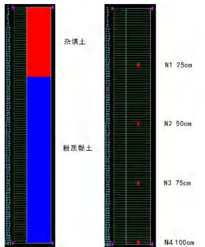
图 5-2-27 土壤污染预测包气带岩性分布及观测点分布图
