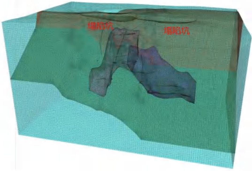
图 5-2-53 III、V 号矿体最终塌陷坑三维透视图
