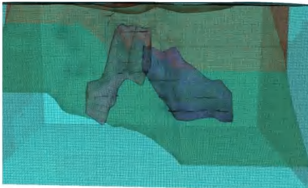
图 5-2-55 III、V 号矿体最终塌陷坑主视图
