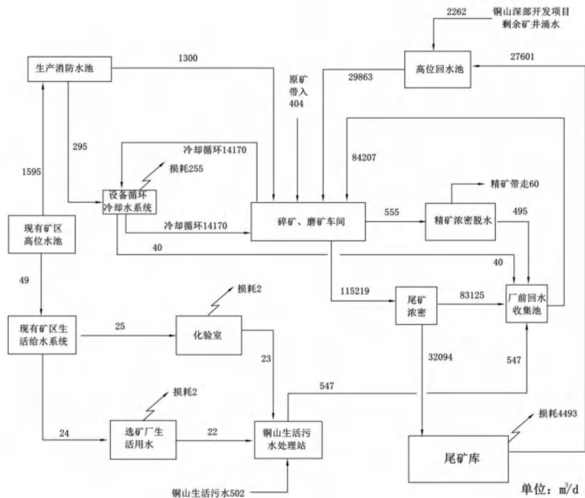
图 3-1-22 在建工程水量平衡图 (冬季) 单位 \text{m}^3/\text{d}
