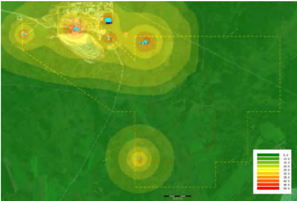
图 5-2-23 矿区噪声贡献值预测图
