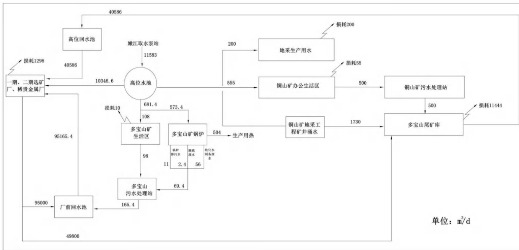
图 3-1-13 矿区现有工程水量平衡图（夏季）
