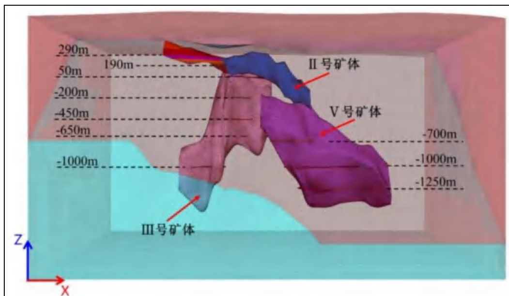
图 5-2-36 铜山矿多矿体协同开采的拉底空间方案图
