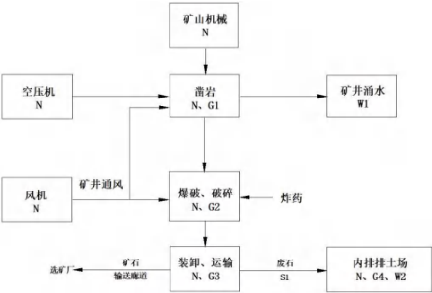
图 3-3-2 采矿工程工艺流程及产污节点图
