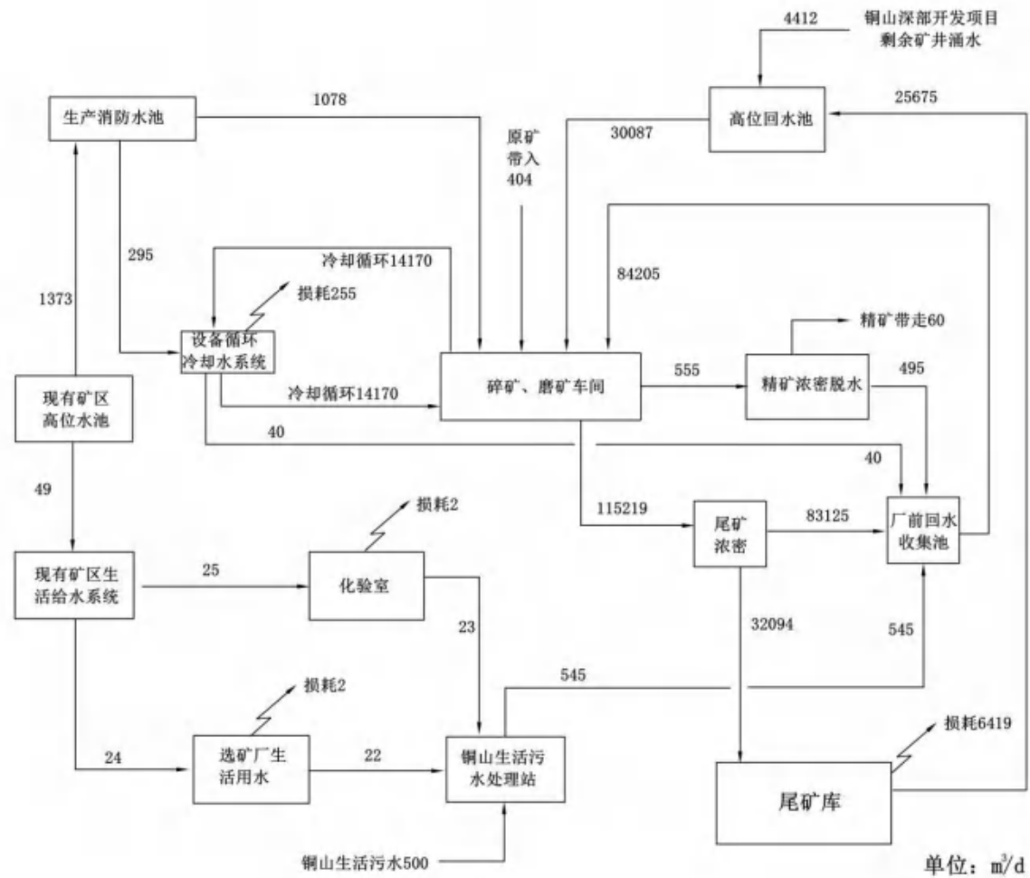
图 3-1-21 在建工程水量平衡图 (夏季) 单位 \text{m}^3/\text{d}
