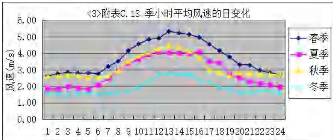
图 4-1-9 季小时平均风速的日变化曲线图
