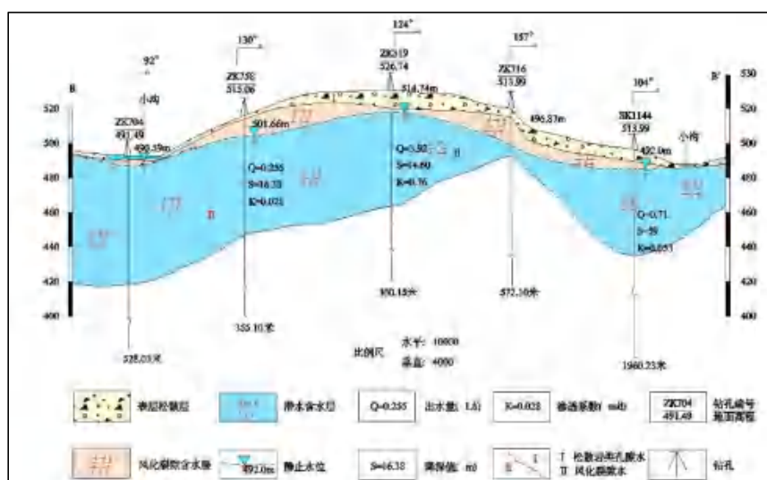
图 5-2-13 矿区地下水含水层剖面图
