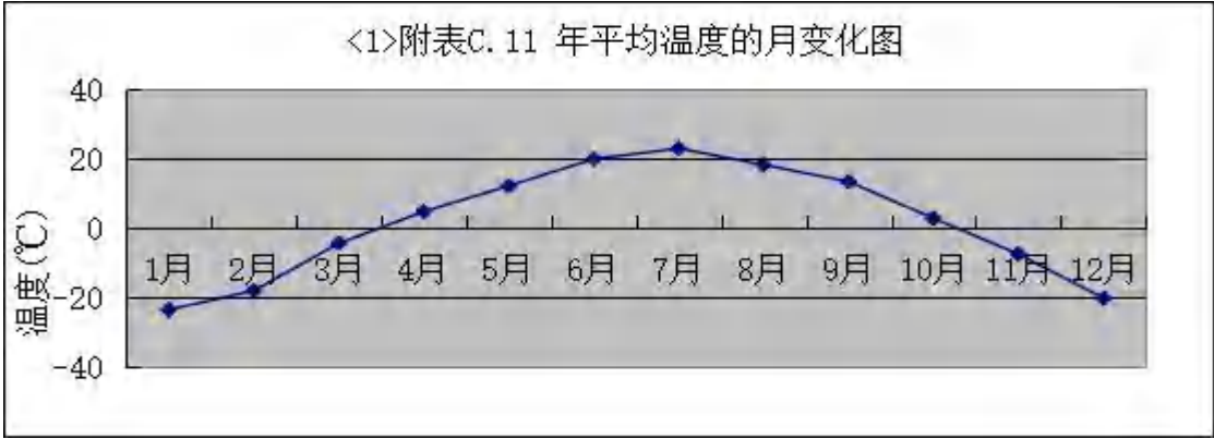
图 4-1-7 年平均温度的月变化曲线图
