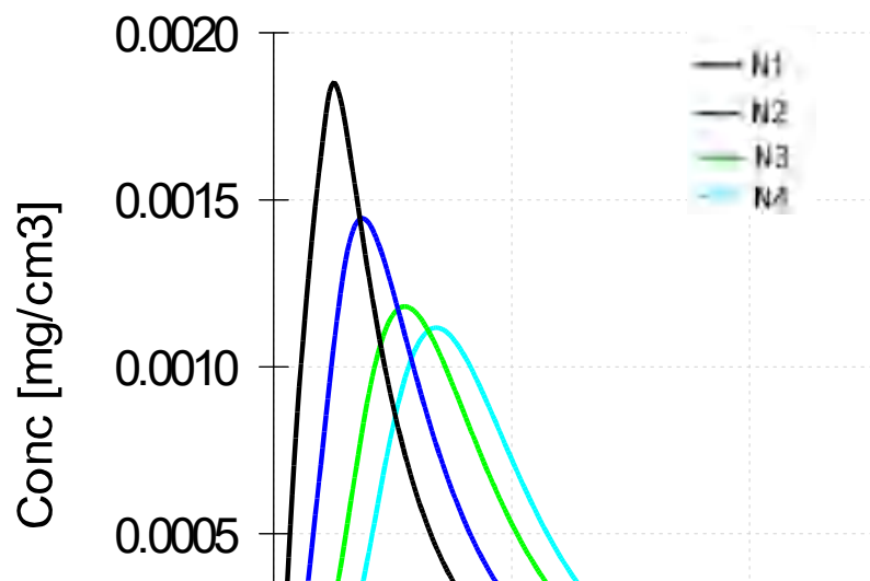
图 5-2-34 泄漏 350d 内地面以下各观测点铅浓度-时间变
