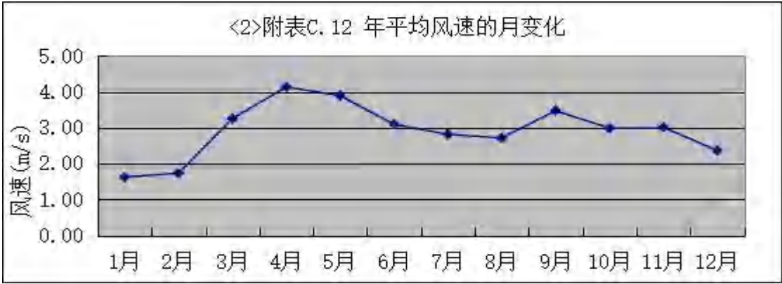
图 4-1-8 年平均风速的月变化曲线
