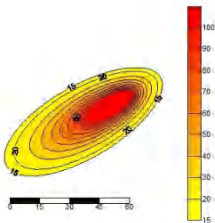
图 5-2-18 非正常状况下 COD 污染晕扩散预测图（1000d）
