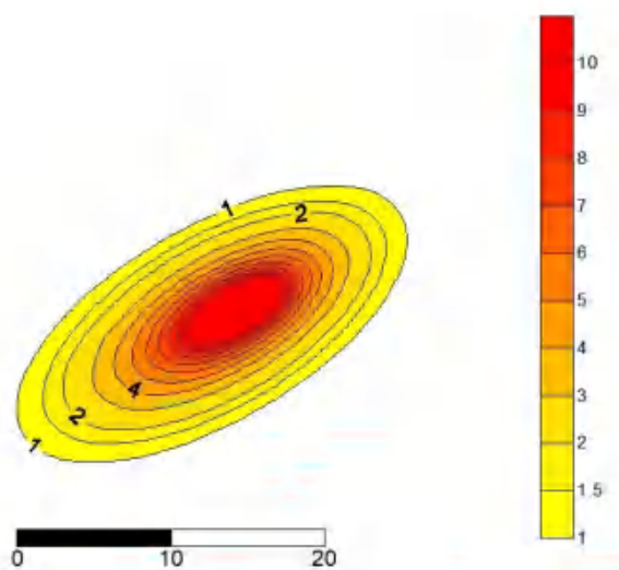
图 5-2-20 非正常状况下氟化物扩散预测图 (100d)
