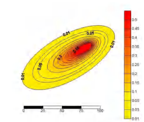
图 5-2-14 非正常状况下铅扩散预测图（100d）
