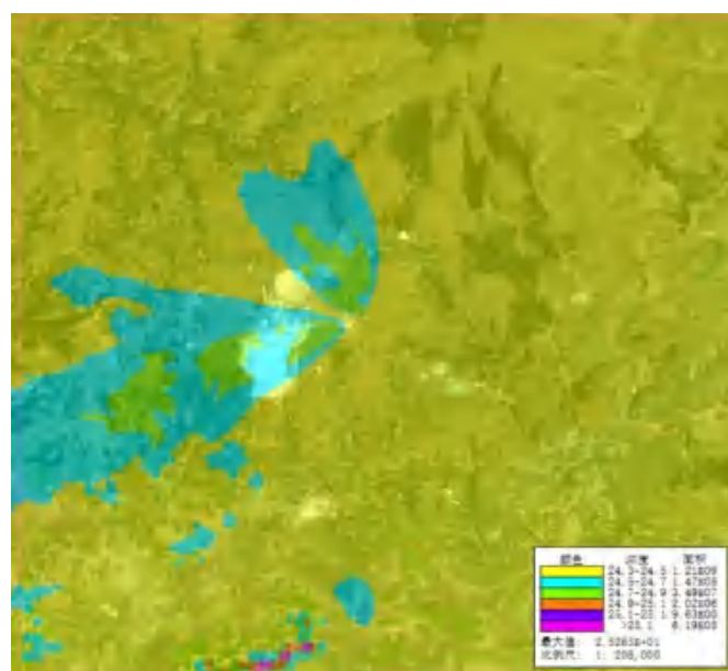
图 5-2-9 本项目 NO 2 保证率日平均质量浓度分布图 (ug/m 3 )
