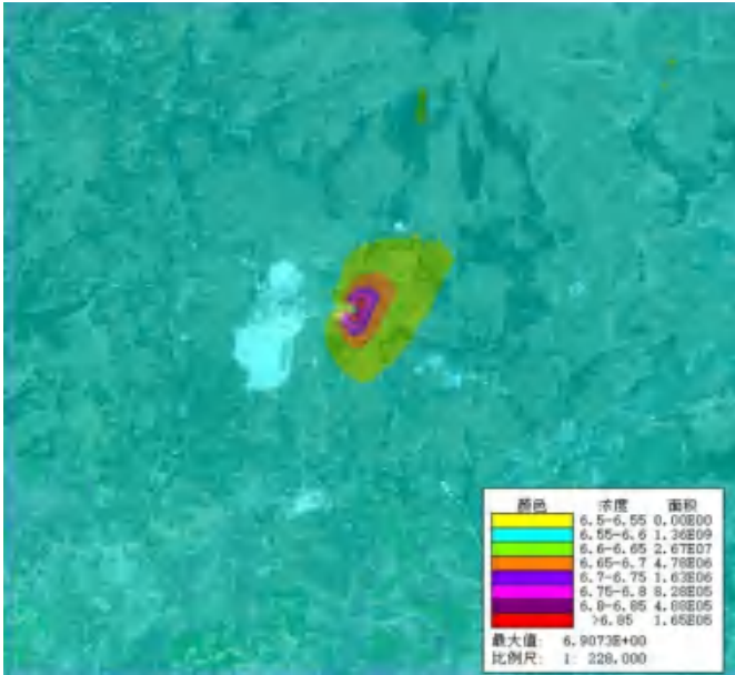
图 5-2-6 本项目 SO 2 年平均质量浓度分布图 (ug/m 3 )
