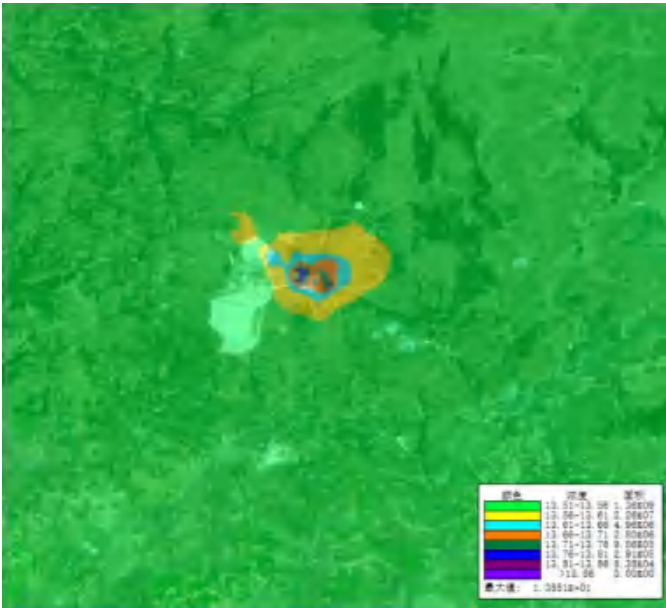
图 5-2-4 本项目 PM 2.5 年平均质量浓度分布图 (ug/m 3 )
