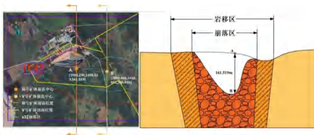
图 5-2-48 沿矿体走向III号矿体塌陷坑中心剖面图
